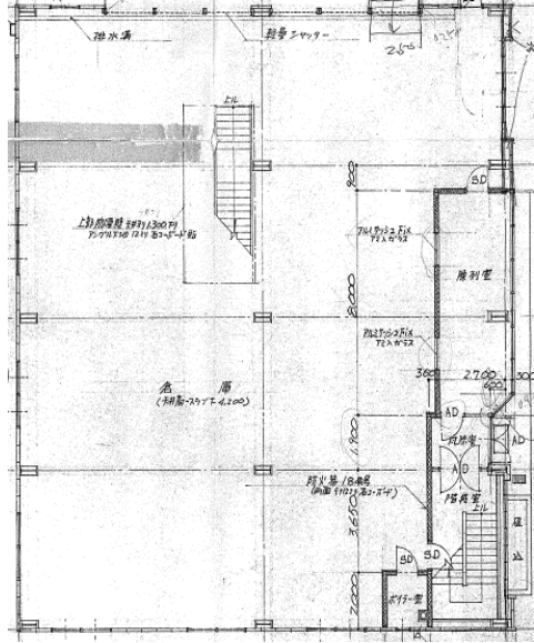
1階: 130.530坪
