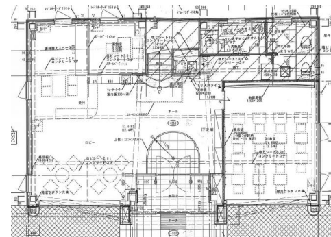
1階図面
