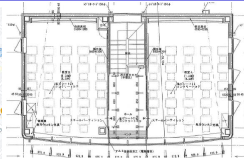
3階図面
