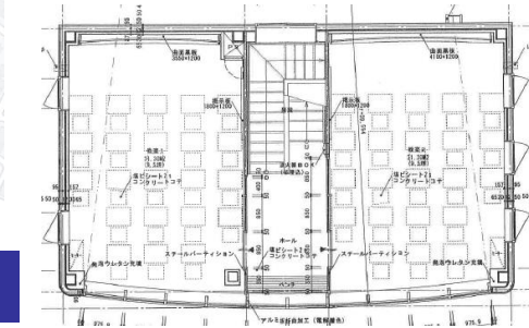
2階図面
