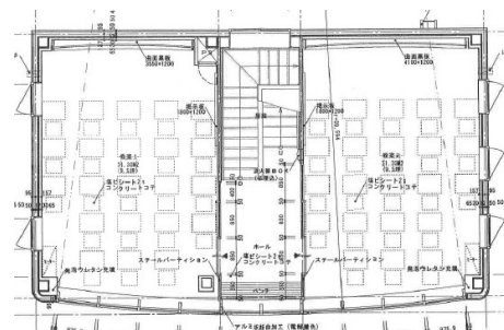
2階図面
