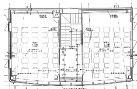
2階図面
