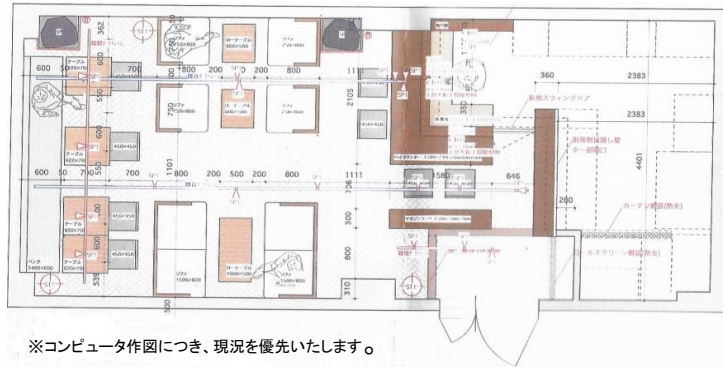
内装
