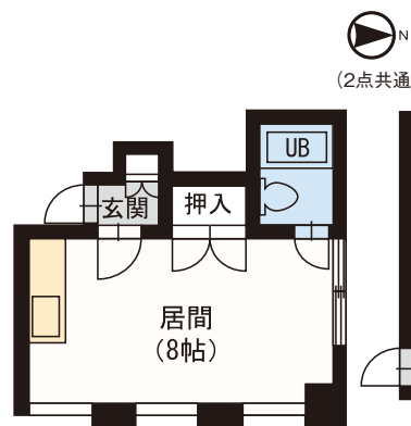
●1R / 21.50㎡
